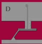
Canto Oculto con Perfil T24
