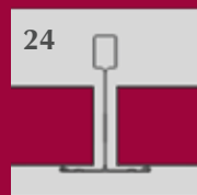
Canto Recto con Perfil T24
