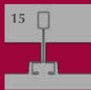
Canto Semioculto con Perfil Fineline T15
